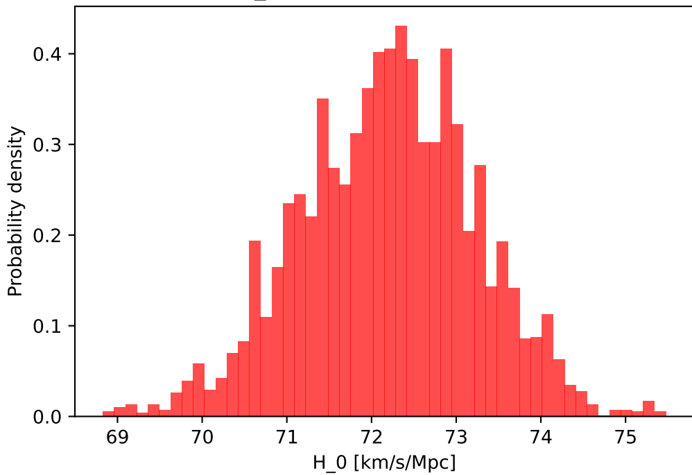
H 0 posterior - USF model
