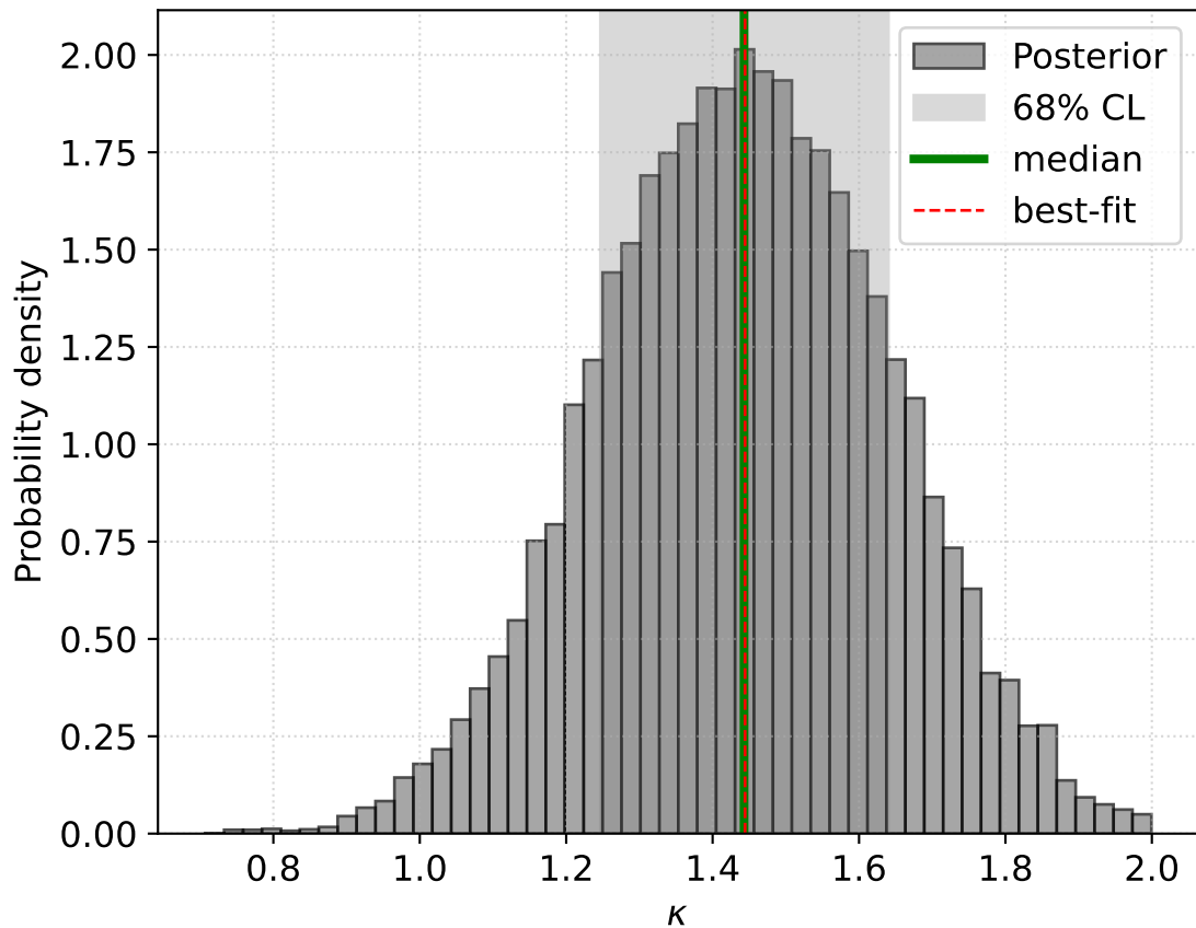
Posterior distribution of \kappa (USF)
