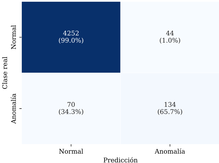
Matriz de Confusión — Isolation Forest (testeo)
