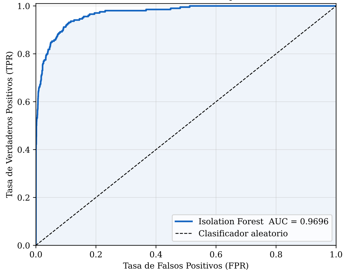
Curva ROC — Isolation Forest (conjunto de testeo)
