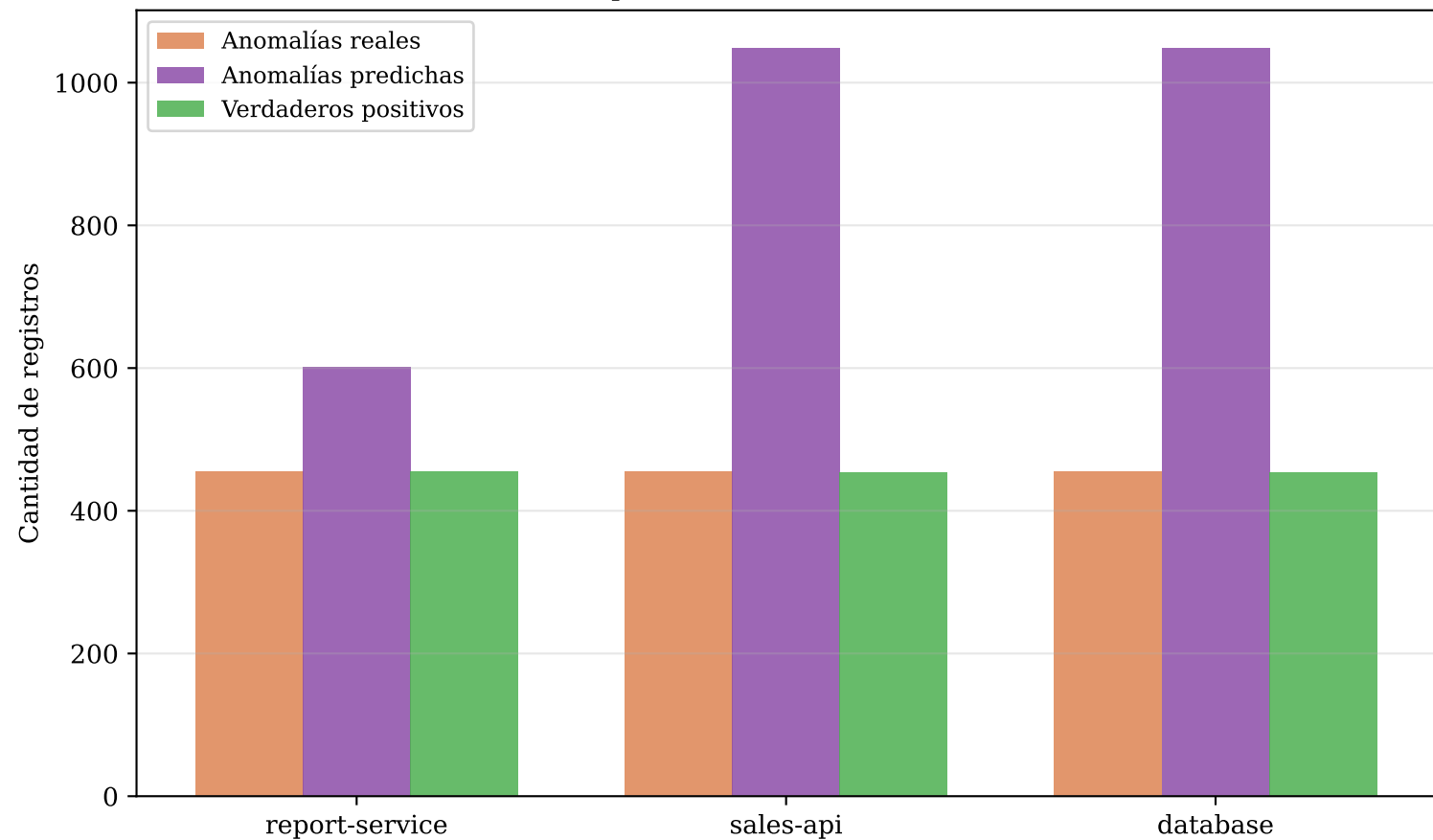
Detección por servicio — Local Outlier Factor
