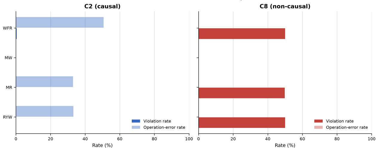
图 7. C2 与 C8 在 S4 下的对照：写/读关注与读偏好相同，唯一差异是因果会话。
