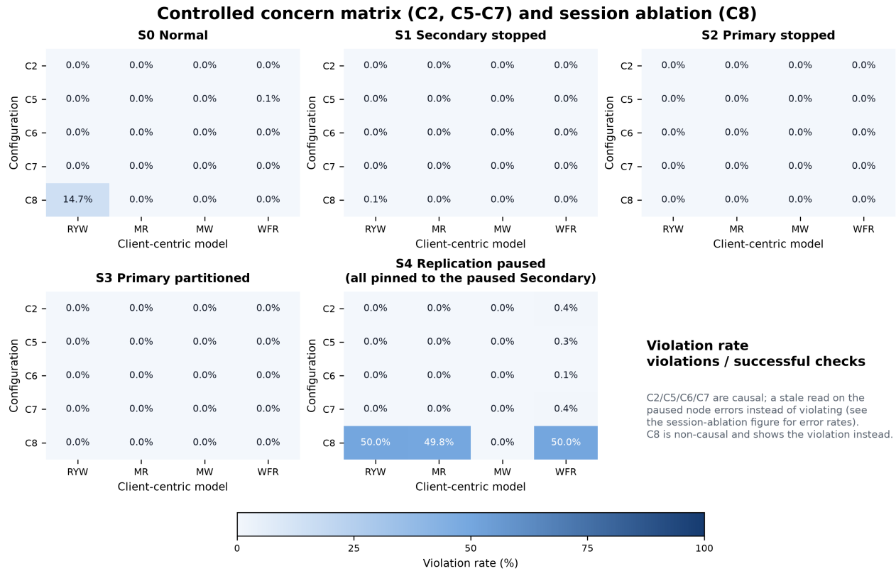
图 6. C2、C5-C8 在 S0-S4 下的违例率矩阵；S4 中所有配置读取同一个被暂停应用 oplog 的 Secondary。
