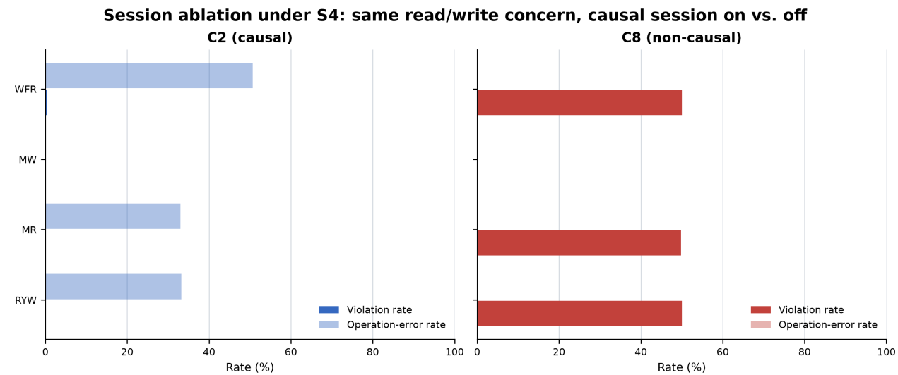
图 7. C2 与 C8 在 S4 下的对照：写/读关注与读偏好相同，唯一差异是因果会话。
