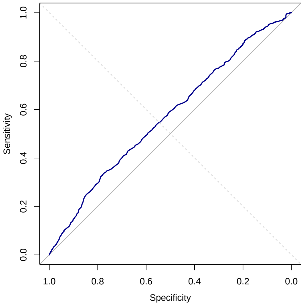
ROC Curve (AUC = 0.571)
