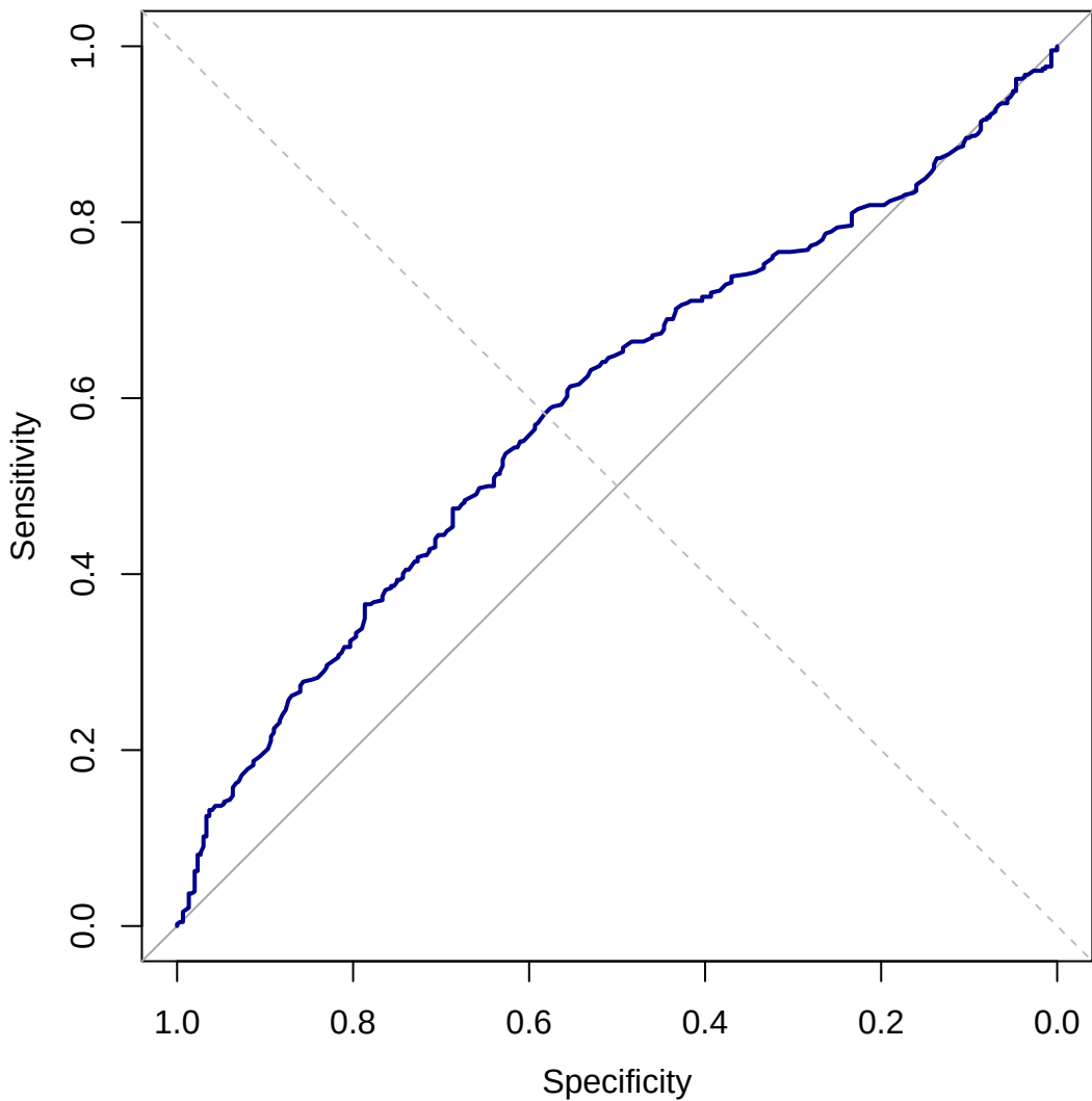
ROC Curve (AUC = 0.592)
