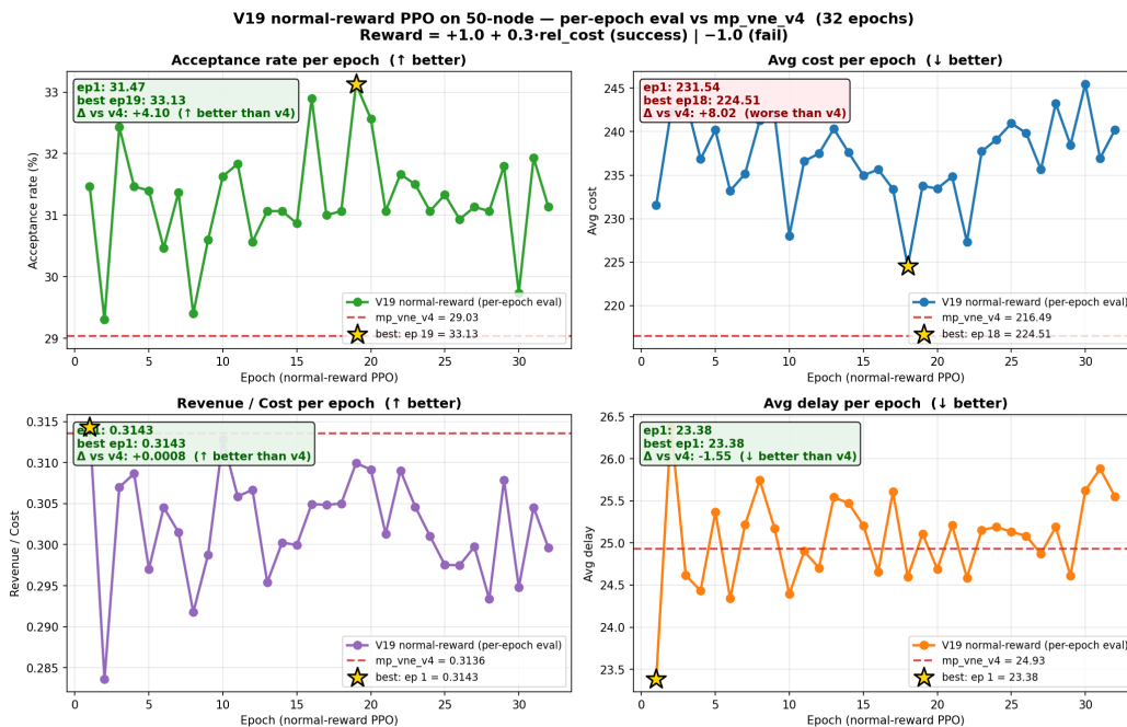
Hình 5.1: So sánh CARL-VNE (theo từng epoch) với baseline MP-VNE-V4 trên kịch bản 50 nút, bốn độ đo: tỷ lệ chấp nhận, chi phí, R/C, độ trễ.
