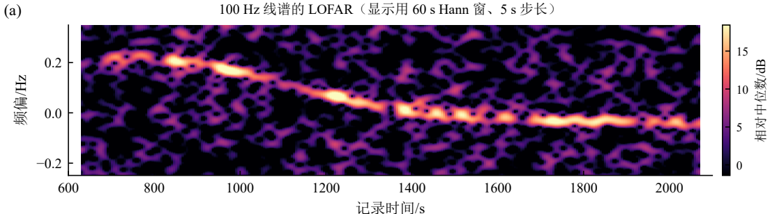
100 Hz 线谱的 LOFAR (显示用 60 s Hann 窗、5 s 步长)
