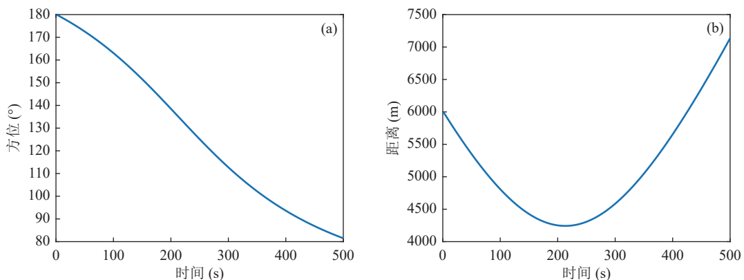
图11 目标方位和距离随时间变化情况 (a) 目标方位; (b) 目标距离
