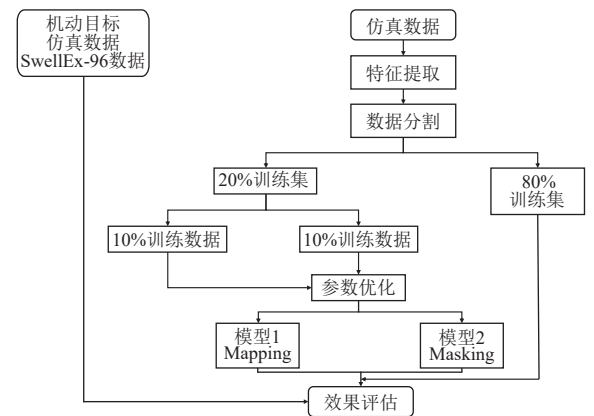
图 4 基于深度学习的水声线谱增强流程图
