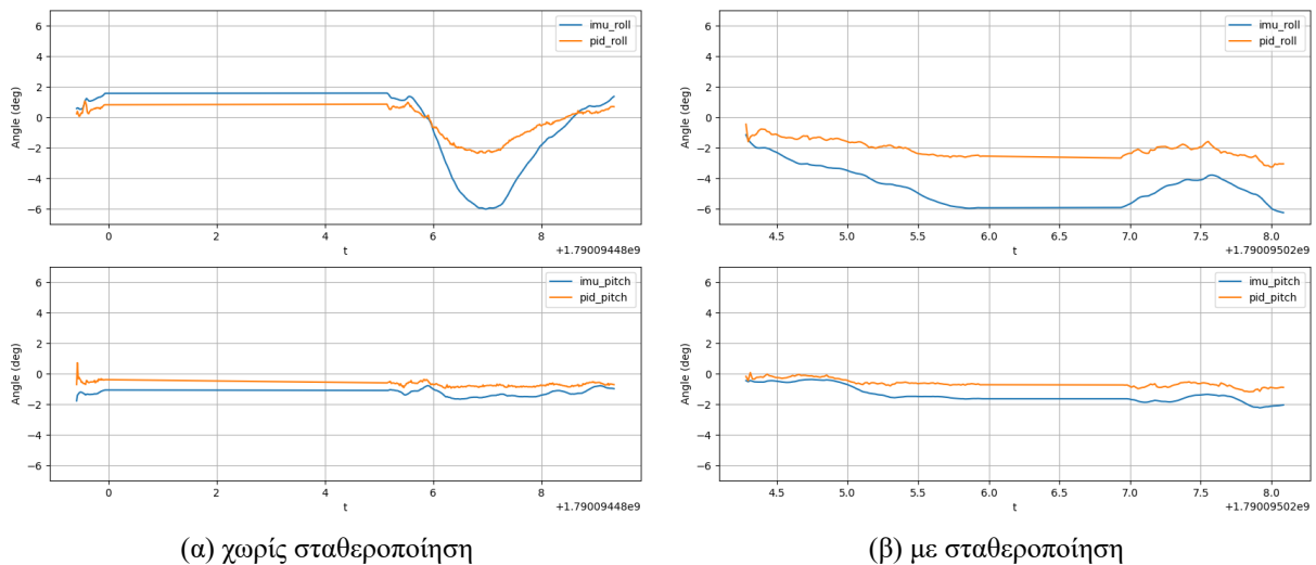
Σχήμα 7.6: Γωνίες roll και pitch για το ίδιο βάδισμα trot προς τα εμπρός. (α) Με τα κέρδη του ελεγκτή μηδενισμένα, οπότε η διόρθωση δεν εφαρμόζεται στα πέλματα. (β) Με τον ελεγκτή ενεργό και τα κέρδη του Πίνακα 4.3
