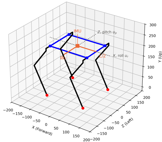
Σχήμα 4.9: (α) Θέση του IMU και αποστάσεις W_f και L/2 της (4.30). (β) Πλάγια όψη σε κεκλιμένο έδαφος: με τη διόρθωση \Delta y_i το σώμα παραμένει οριζόντιο, ενώ με διακεκομμένη γραμμή φαίνεται το σώμα χωρίς αντιστάθμιση. Κατά το πρότυπο του Σχήματος 4 του [24]
