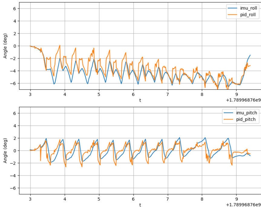
Σχήμα 6.16: Δείγμα του γραφήματος που παράγει η pid_plotter.py στο τέλος κάθε εκτέλεσης, από ένα τυχαίο πέρασμα. Πάνω το roll και κάτω το pitch, με τη μέτρηση του αισθητήρα και την έξοδο του ελεγκτή σε κοινό άξονα
