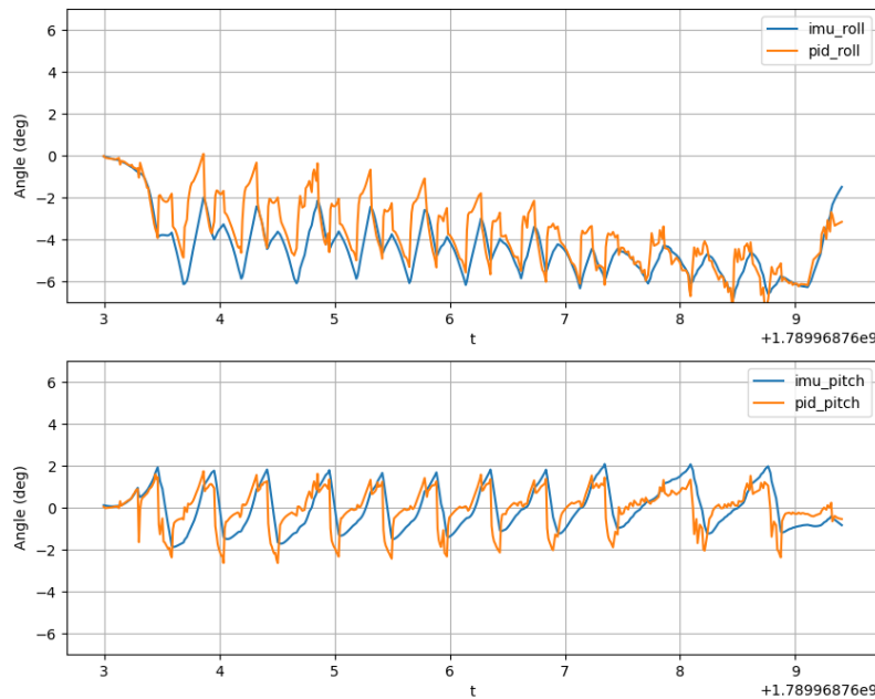
Σχήμα 7.3: Γωνίες roll και pitch στην προσομοίωση, για ταυτόχρονη μετατόπιση προς \lambda = 45^\circ με v = 0,30 m/s και στροφή με \omega = 0,30 rad/s
