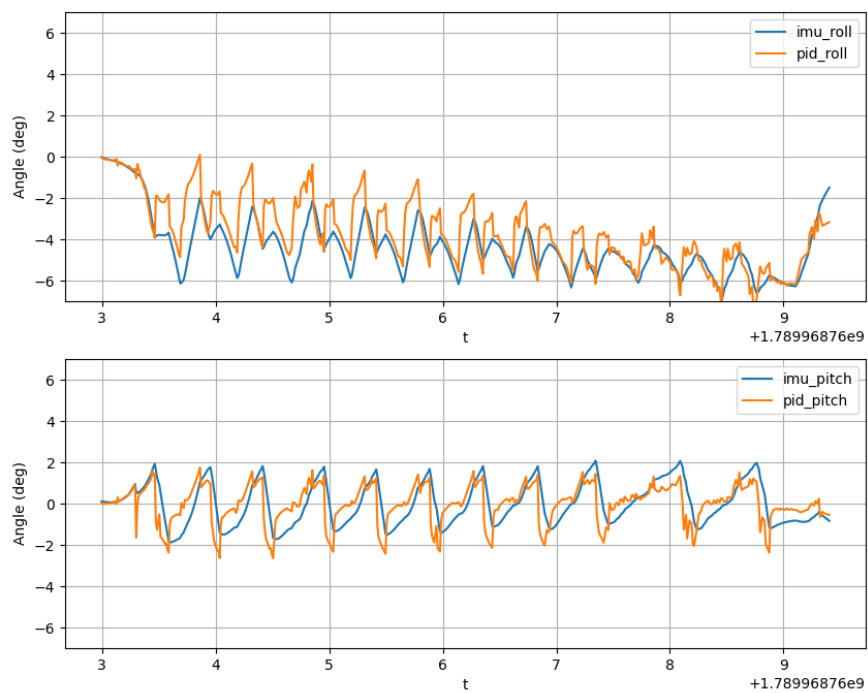
Σχήμα 6.16: Δείγμα του γραφήματος που παράγει η log_plotter.py στο τέλος κάθε εκτέλεσης, από ένα τυχαίο πέρασμα. Πάνω το roll και κάτω το pitch, με τη μέτρηση του αισθητήρα και την έξοδο του ελεγκτή σε κοινό άξονα
