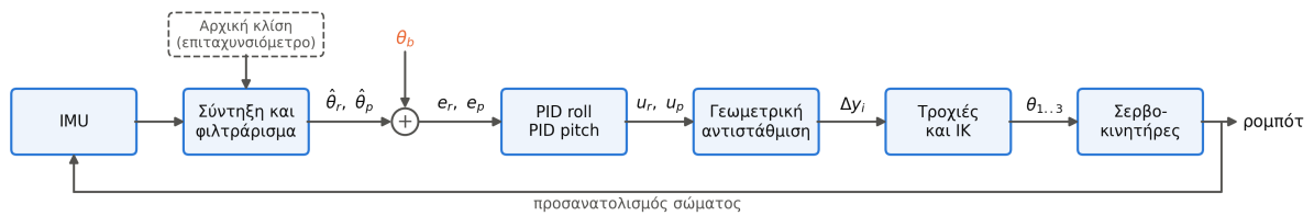
Σχήμα 4.8: Βρόχος ελέγχου σταθεροποίησης προσανατολισμού
