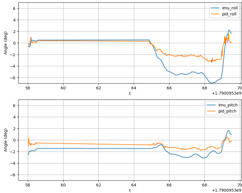
Σχήμα 7.5: Γωνίες roll και pitch στο πραγματικό ρομπότ, για ταυτόχρονη μετατόπιση και στροφή, δηλαδή στην περίπτωση που τα δύο διανύσματα βήματος συντίθενται κατά την (4.25)
