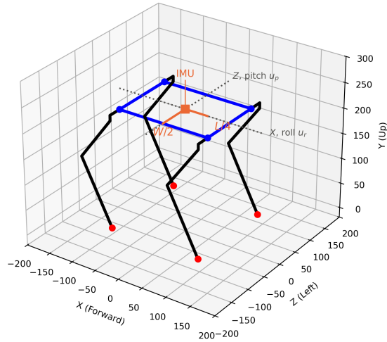
Σχήμα 4.9: (α) Θέση του IMU και αποστάσεις W/2 και L/4 της (4.30). (β) Πλάγια όψη σε κεκλιμένο έδαφος: με τη διόρθωση \Delta y_i το σώμα παραμένει οριζόντιο, ενώ με διακεκομμένη γραμμή φαίνεται το σώμα χωρίς αντιστάθμιση. Κατά το πρότυπο του Σχήματος 4 του [24]
