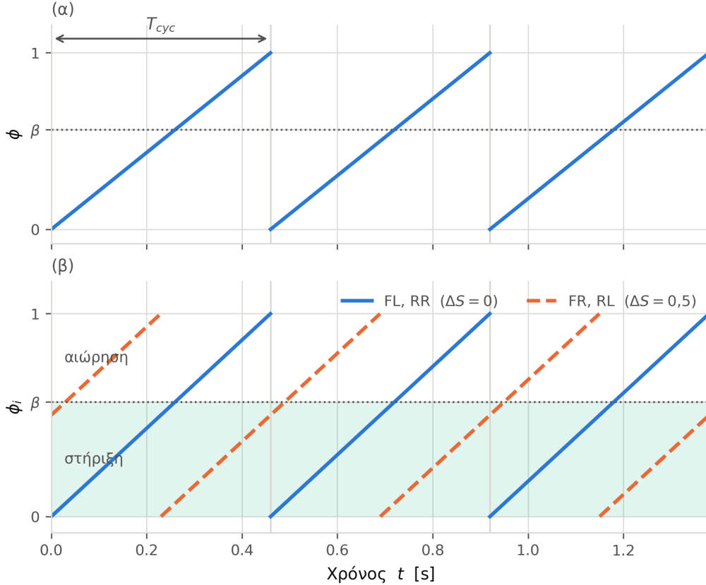
Σχήμα 4.4: Το πριονωτό σήμα της φάσης για T_{cyc} = 0,46 s και \beta = 0,565 . (α) Η καθολική φάση \phi της (4.15). (β) Οι φάσεις \phi_i των ποδιών της (4.16) για το βάδισμα trot: τα δύο διαγώνια ζεύγη διαφέρουν κατά μισό κύκλο, ενώ κάθε πόδι βρίσκεται σε στήριξη όσο \phi_i < \beta
