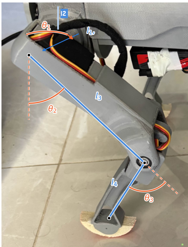
Σχήμα 3.2: Οι τρεις γωνίες άρθρωσης και τα τέσσερα μήκη συνδέσμων, σημειωμένα στο εμπρός αριστερό σκέλος του ρομπότ. Οι γωνίες \theta_2 και \theta_3 μετρώνται από τις διακεκομμένες διευθύνσεις αναφοράς, ενώ η \theta_1 περιστρέφει ολόκληρο το επίπεδο του σκέλους γύρω από τον άξονα του ώμου. Οι μετατοπίσεις l_1 και l_2 βρίσκονται στο εσωτερικό του ώμου. Λόγω της προοπτικής, οι ενδείξεις δείχνουν ποιο μέγεθος είναι ποιο και όχι πραγματικές αναλογίες
