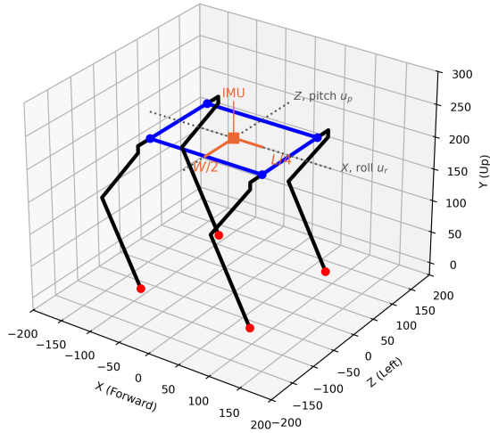
Σχήμα 4.9: (α) Θέση του IMU και αποστάσεις W/2 και L/4 της (4.30). (β) Πλάγια όψη σε κεκλιμένο έδαφος: με τη διόρθωση \Delta y_i το σώμα παραμένει οριζόντιο, ενώ με διακεκομμένη γραμμή φαίνεται το σώμα χωρίς αντιστάθμιση. Κατά το πρότυπο του Σχήματος 4 του [24]
