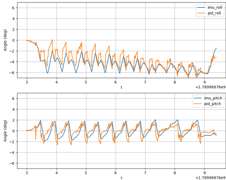
Σχήμα 7.3: Γωνίες roll και pitch στην προσομοίωση, για ταυτόχρονη μετατόπιση προς \lambda = 45^\circ με v = 0,30 m/s και στροφή με \omega = 0,30 rad/s
