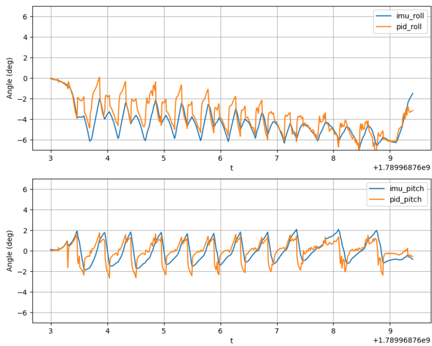
Σχήμα 6.16: Δείγμα του γραφήματος που παράγει η log_plotter.py στο τέλος κάθε εκτέλεσης, από ένα τυχαίο πέρασμα. Πάνω το roll και κάτω το pitch, με τη μέτρηση του αισθητήρα και την έξοδο του ελεγκτή σε κοινό άξονα
