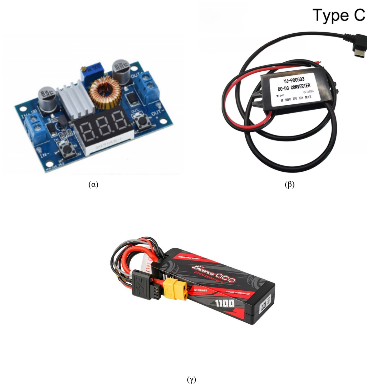
Σχήμα 6.8: (α) Ο μετατροπέας υποβιβασμού τάσης για τροφοδοσία των οδηγών servo (β) Ο μετατροπέας υποβιβασμού τάσης για τροφοδοσία του Raspberry Pi 5 (γ) Η LiPo μπαταρία για τροφοδοσία όλης της πλατφόρμας
