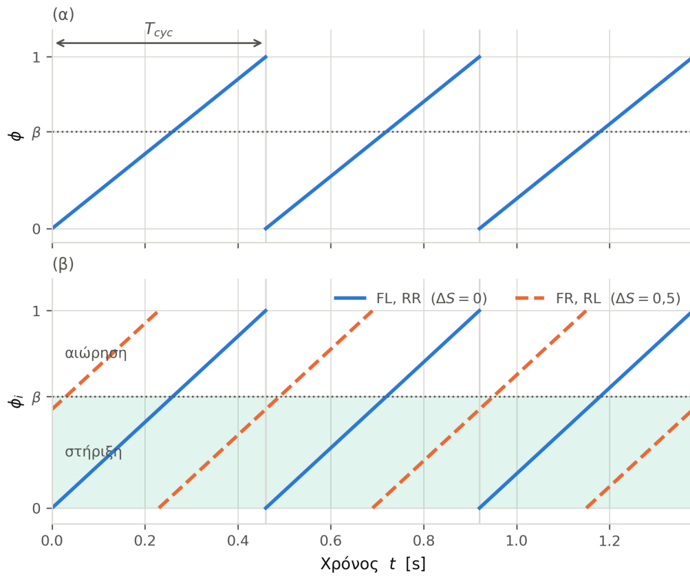
Σχήμα 4.4: Το πριονωτό σήμα της φάσης για T_{cyc} = 0,46 s και \beta = 0,565 . (α) Η καθολική φάση \phi της (4.14). (β) Οι φάσεις \phi_i των ποδιών της (4.15) για το βάδισμα trot: τα δύο διαγώνια ζεύγη διαφέρουν κατά μισό κύκλο, ενώ κάθε πόδι βρίσκεται σε στήριξη όσο \phi_i < \beta
