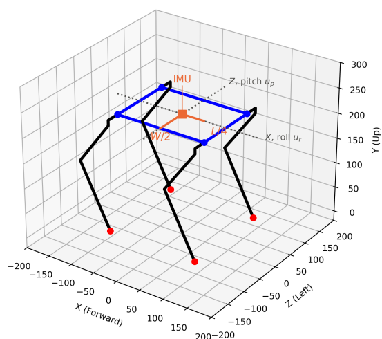
Σχήμα 4.9: (α) Θέση του IMU και αποστάσεις W/2 και L/4 της (4.29). (β) Πλάγια όψη σε κεκλιμένο έδαφος: με τη διόρθωση \Delta y_i το σώμα παραμένει οριζόντιο, ενώ με διακεκομμένη γραμμή φαίνεται το σώμα χωρίς αντιστάθμιση. Κατά το πρότυπο του Σχήματος 4 του [24]
