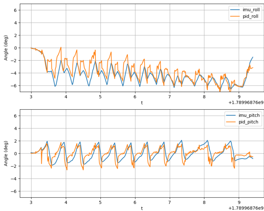
Σχήμα 6.18: Δείγμα του γραφήματος που παράγει η log_plotter.py στο τέλος κάθε εκτέλεσης, από ένα τυχαίο πέρασμα. Πάνω το roll και κάτω το pitch, με τη μέτρηση του αισθητήρα και την έξοδο του ελεγκτή σε κοινό άξονα
