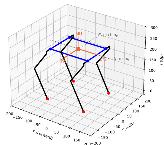
Σχήμα 4.9: (α) Θέση του IMU και αποστάσεις W_f και L/2 της (4.30). (β) Πλάγια όψη σε κεκλιμένο έδαφος: με τη διόρθωση \Delta y_i το σώμα παραμένει οριζόντιο, ενώ με διακεκομμένη γραμμή φαίνεται το σώμα χωρίς αντιστάθμιση. Κατά το πρότυπο του Σχήματος 4 του [24]
