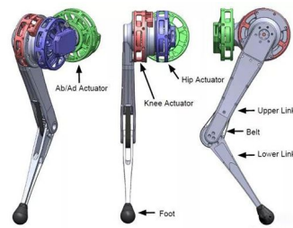
Σχήμα 2.4: Proximal actuation στον ώμο (φιλοσοφία Unitree/MIT Cheetah)
