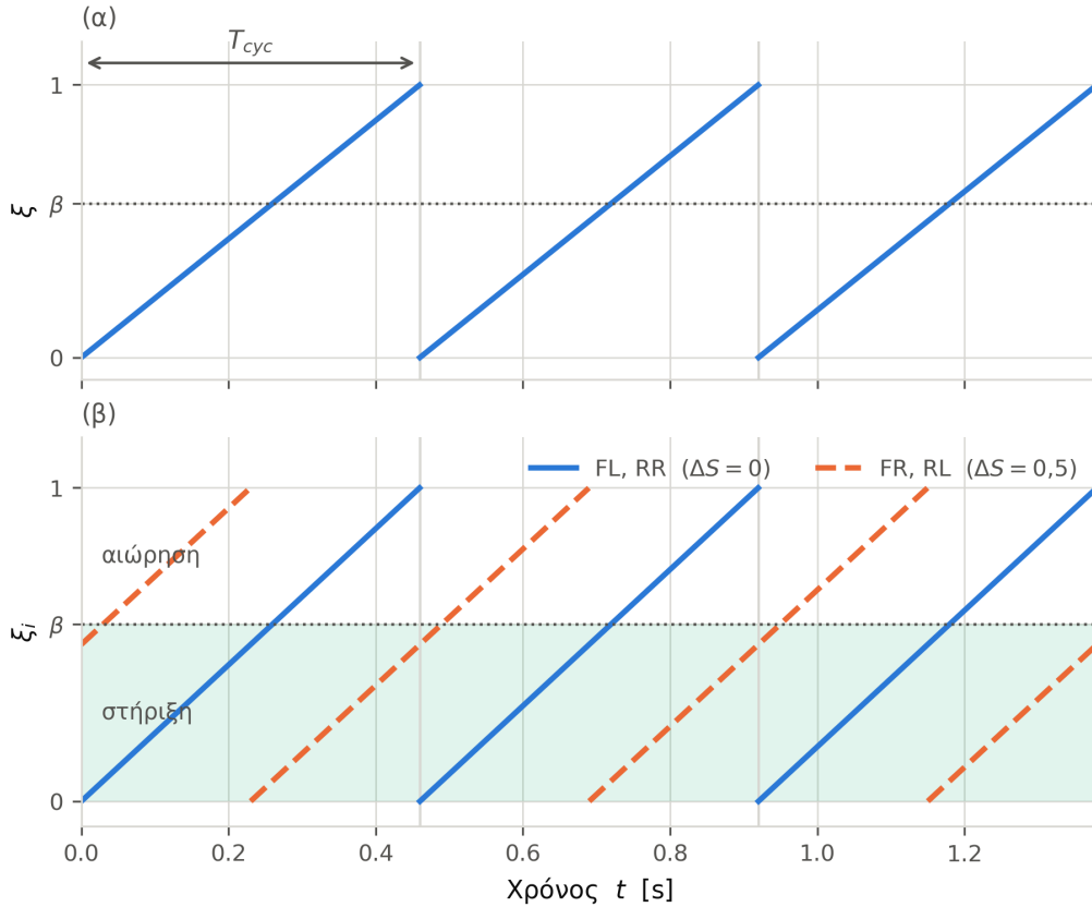
Σχήμα 4.4: Το πριονωτό σήμα της φάσης για T_{cyc} = 0,46 s και \beta = 0,565 . (α) Η καθολική φάση \xi της (4.15). (β) Οι φάσεις \xi_i των ποδιών της (4.16) για το βήδισμα trot: τα δύο διαγώνια ζεύγη διαφέρουν κατά μισό κύκλο, ενώ κάθε πόδι βρίσκεται σε στήριξη όσο \xi_i < \beta
