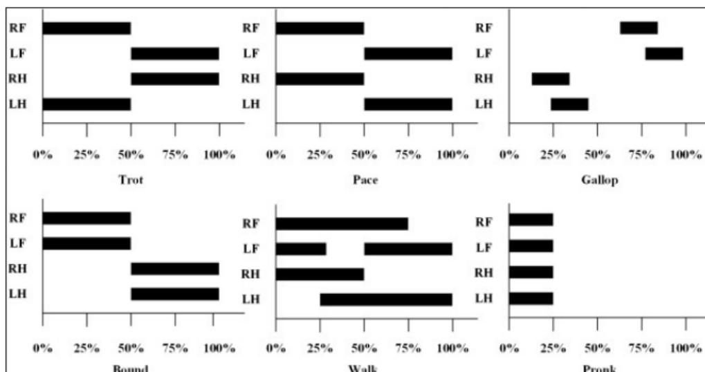
Σχήμα 2.3: Διάγραμμα φάσεων βαδίσματος (gait diagram) για trot, pace, gallop, bound, walk και pronk
