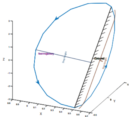
Σχήμα 2.9: Ελλειπτική τροχιά ποδιού. Πηγή: [24]
