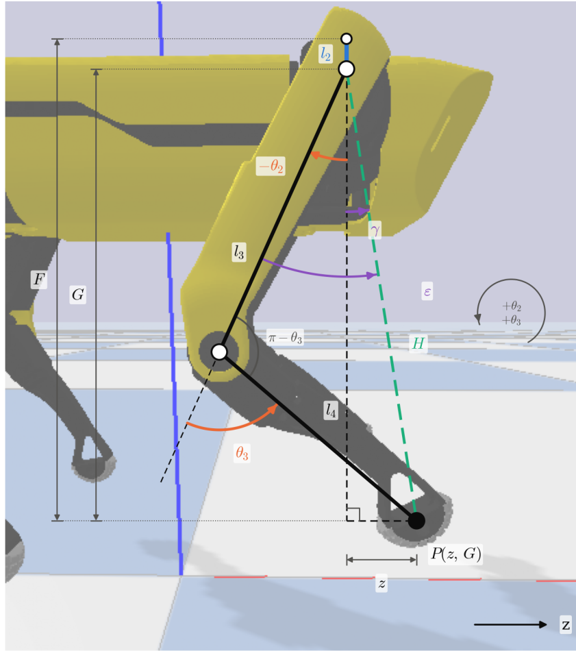
Σχήμα 3.4: Αντίστροφη κινηματική στο επίπεδο του σκέλους, σημειωμένη πάνω σε πλευρικό στιγμιότυπο της προσομοίωσης PyBullet. Το τρίγωνο με πλευρές l_3 , l_4 και H δίνει την \theta_3 της (3.14), ενώ η \theta_2 αναλύεται στις γωνίες \gamma και \varepsilon της (3.16), με \theta_2 = \gamma - \varepsilon . Επειδή η \theta_2 είναι αρνητική, στο σχήμα σημειώνεται το μέτρο της, -\theta_2
