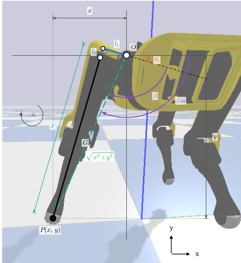
Σχήμα 3.3: Αντίστροφη κινηματική στο εγκάρσιο επίπεδο, δηλαδή στο επίπεδο x - y του ώμου, σημειωμένη πάνω σε στιγμιότυπο της προσομοίωσης PyBullet. Η \theta_1 είναι η κλίση του συνδέσμου l_1 ως προς τον άξονα x και ισχύει \theta_1 = -(\alpha + \beta) της (3.12). Επειδή η \alpha είναι αρνητική, στο σχήμα σημειώνεται το μέτρο της, -\alpha
