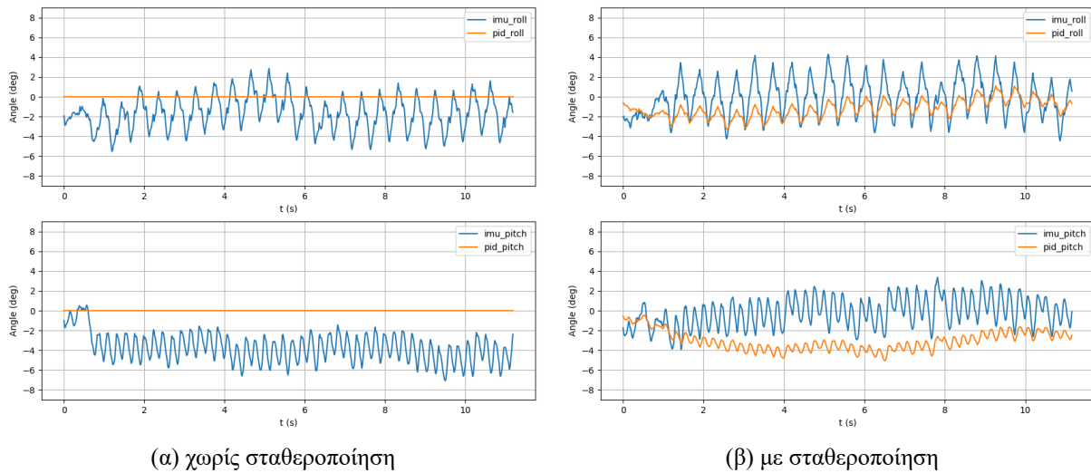
Σχήμα 7.6: Γωνίες roll και pitch για βάδισμα trot προς τα εμπρός. (α) Με μηδενικά κέρδη. (β) Με τον ελεγκτή ενεργό και τα κέρδη του Πίνακα 4.3
