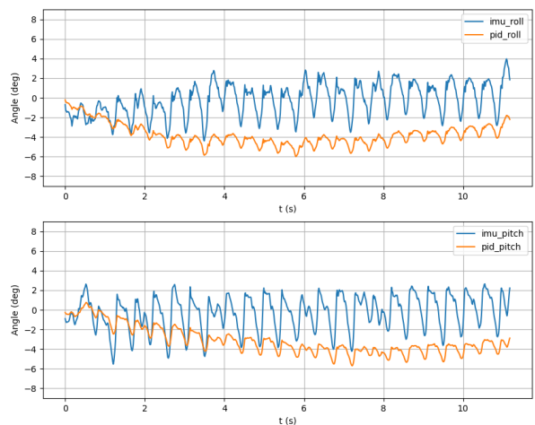
(β) στροφή εν κινήσει
