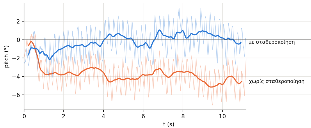
Σχήμα 7.7: Γωνία pitch κατά το βάδισμα εμπρός, χωρίς ελεγκτή και με τον ελεγκτή PI. Με λεπτή γραμμή η μέτρηση και με έντονη η μέση τιμή σε ένα κύκλο βαδίσματος
