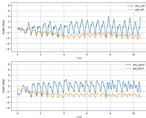
(α) στροφή επί τόπου
