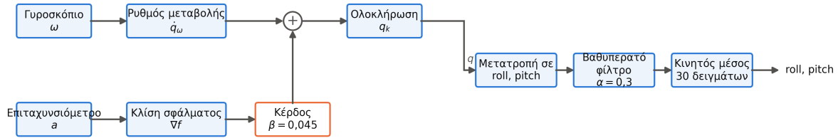
Σχήμα 6.12: Δομή του φίλτρου Madgwick: ο ρυθμός μεταβολής από το γυροσκόπιο διορθώνεται από την κλίση του σφάλματος του επιταχυνσιόμετρου με κέρδος \beta = 0,045
