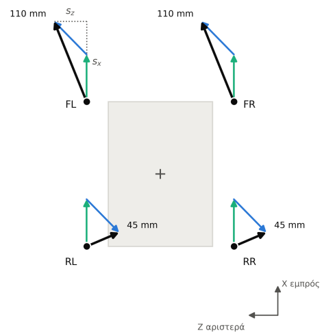
(δ) Γραμμική + στροφή, R = v/\omega = 300 \text{ mm}
