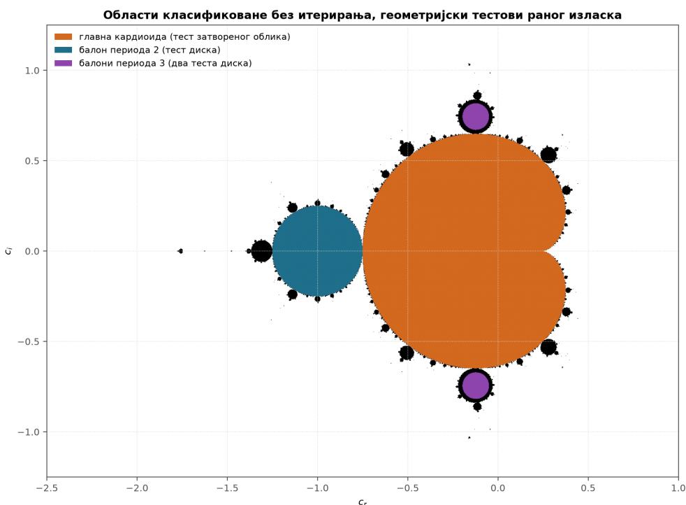
Слика 3.3.1: Три области затвореног облика приказане на рендеру целог кадра Манделбрововог скупа: главна кардиоиду, балон периода 2 и два балона периода 3. Сваком пикселу унутар осенчене области директно се додељује max_iter , без икакве итерације. Свуда другде, укључујући и мање сателитске балоне видљиве дуж границе, и даље се извршава пуна петља.
