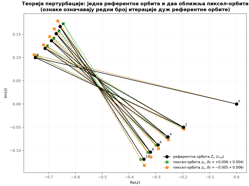
Слика 3.6.1: Стварна референтна орбита у c_{\text{ref}} = -0.75 + 0.1i , тачки „долине морских коњица” коју користи и одељак 6.3.2, заједно са две орбите пиксела удаљене за мало \delta c . Све три орбите остају близу једна другој за приказане итерације, што је управо оно што омогућава да \delta_n буде представљено у обичном f64, док сама Z_n носи проширену прецизност.
