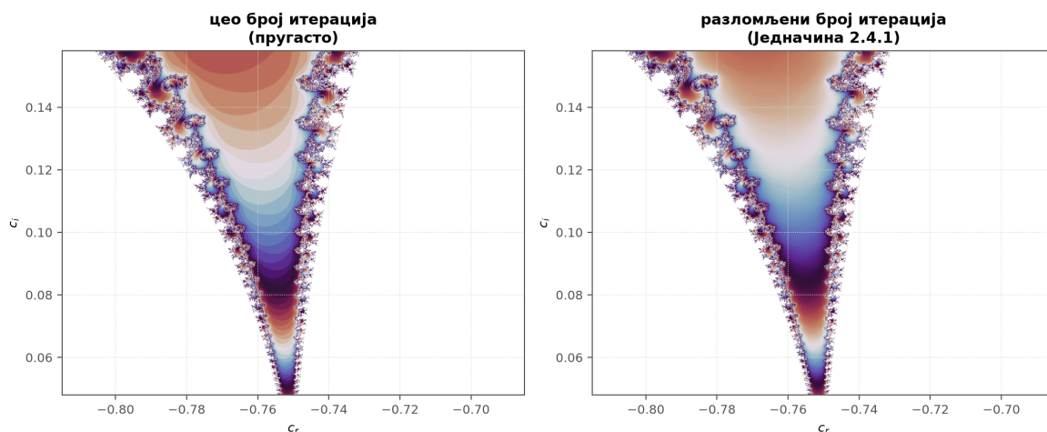
Слика 2.4.1: Иста гранична област обојена сировим целобројним бројем итерација и глатким бројем из једначине 2.4.1. Прстенови на левој слици настају понављањем палете једном по целој итерацији. Десна слика пролази кроз исту палету, али интерполира унутар сваког прстена.
