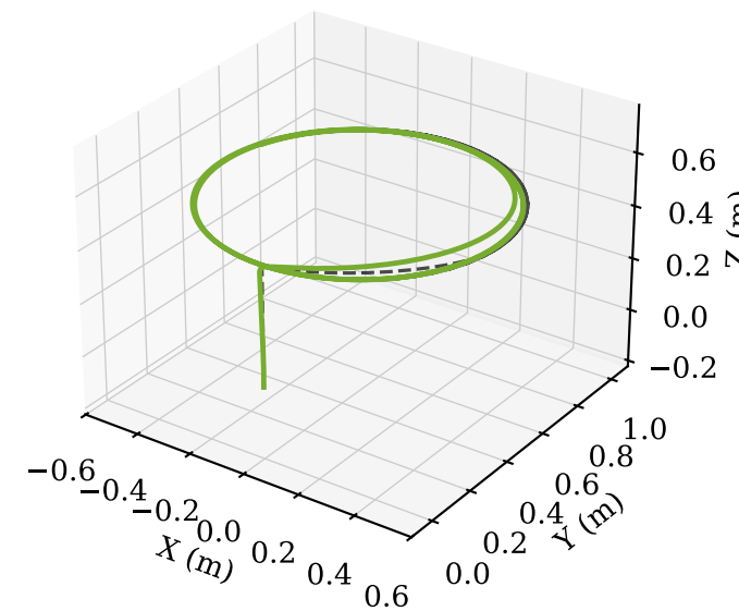
PID+MPC
