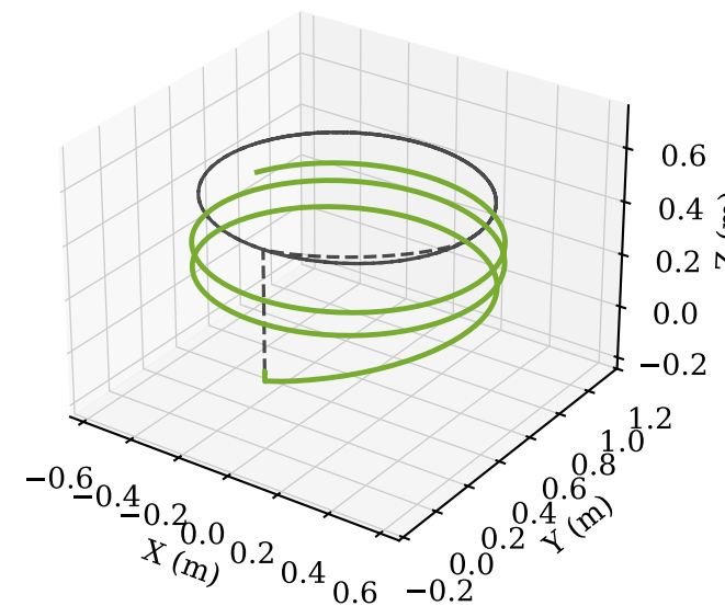
PID+MPC
