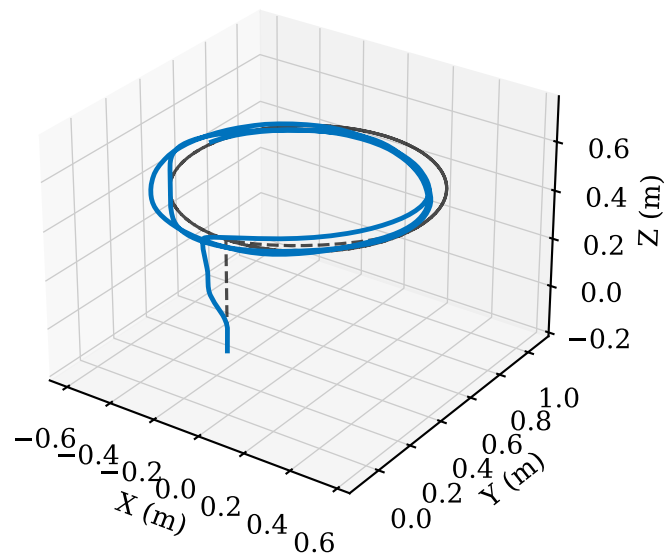
MPC
