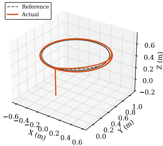
PID
