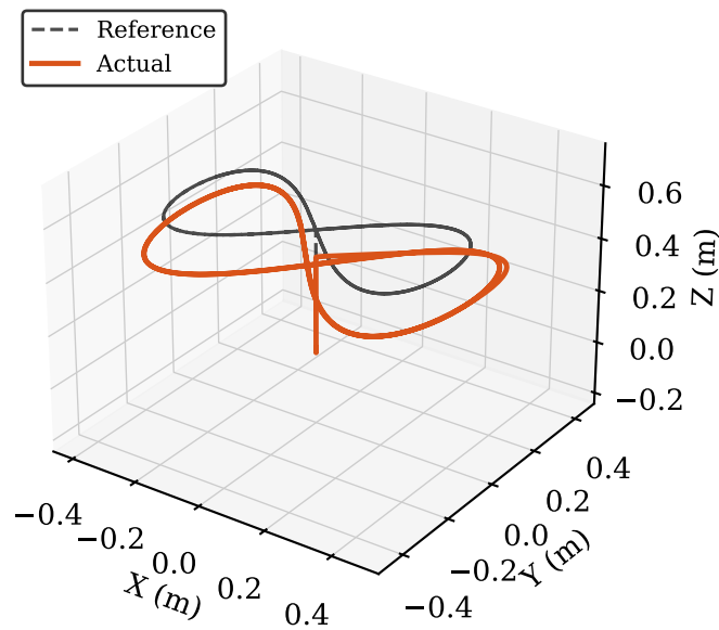
PID
