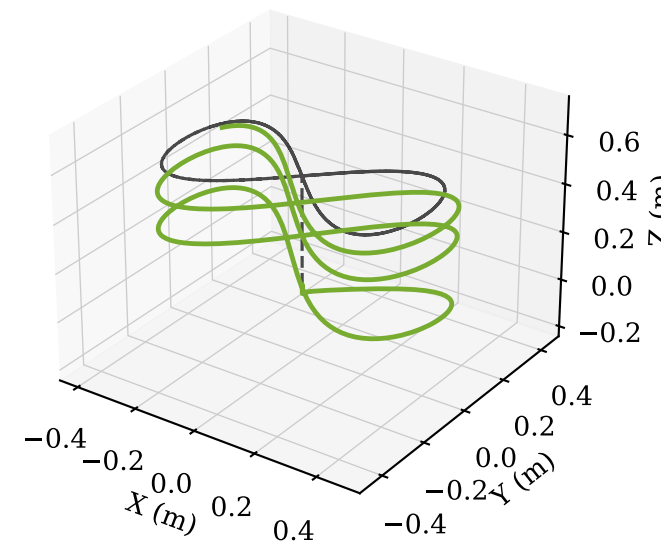
PID+MPC
