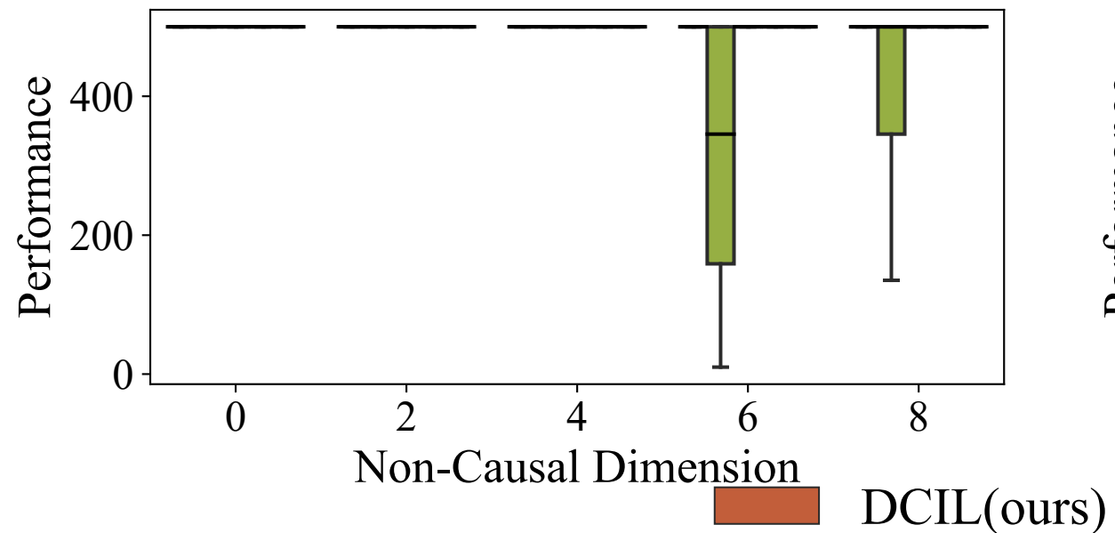
CartPole-v1
