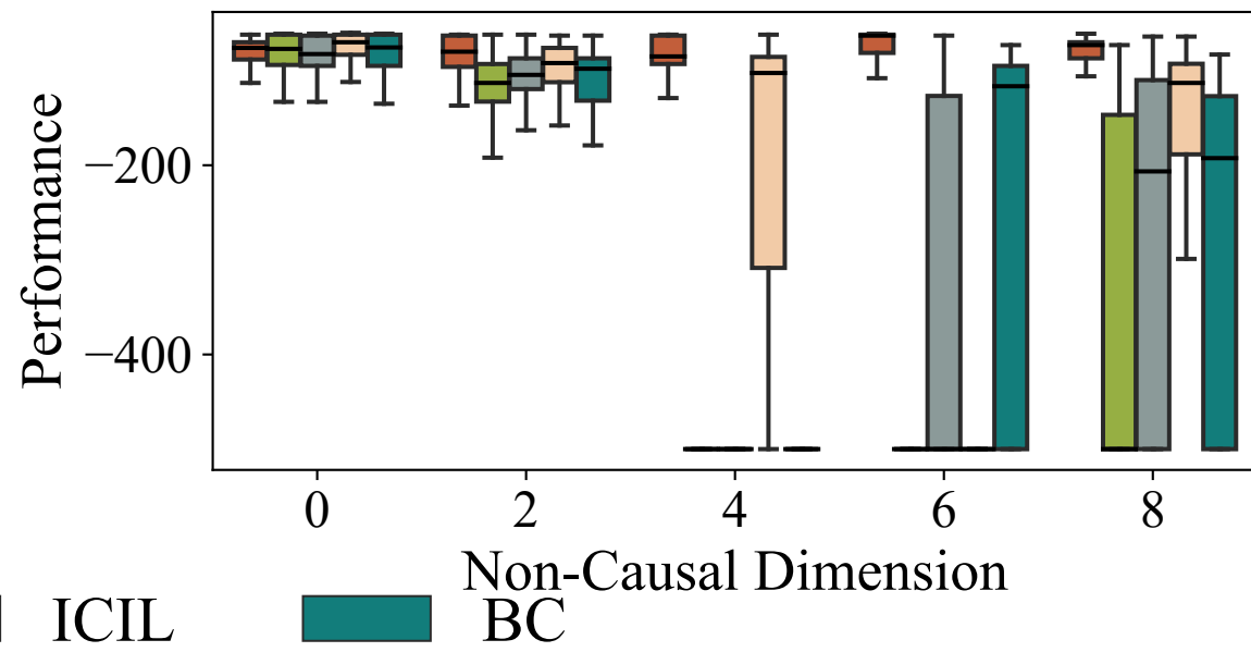
Acrobot-v1
