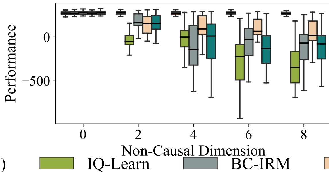
LunarLander-v2
