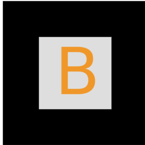
dopamina
