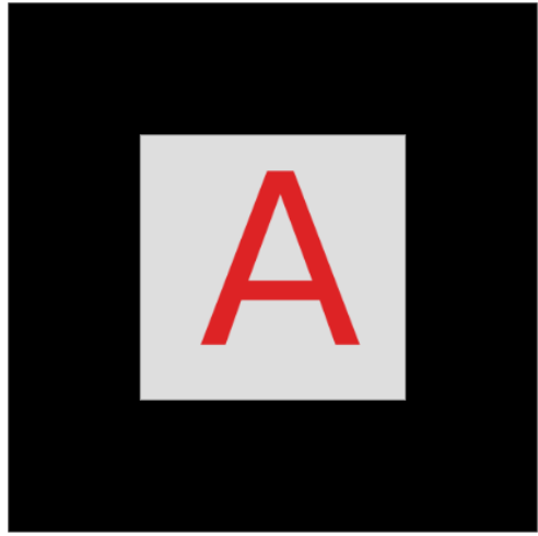
E. iónico
