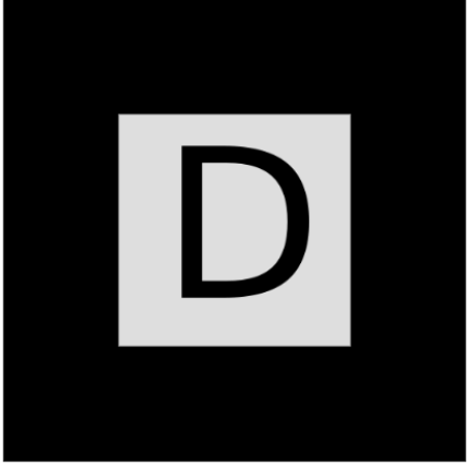
grafito
