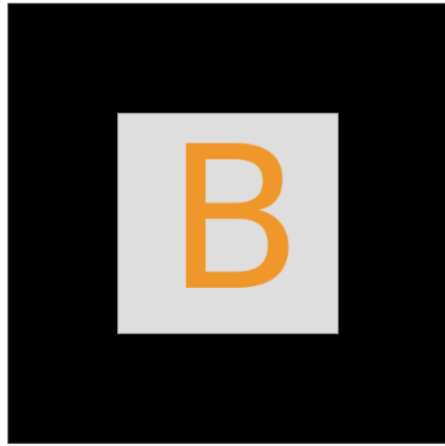
E. Covalente simple
