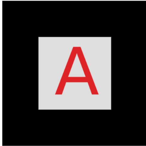
célula
