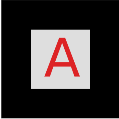
molécula
