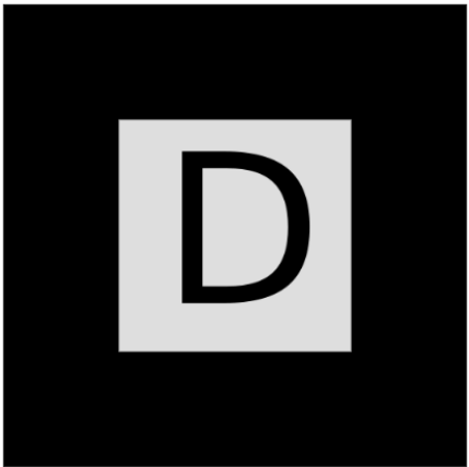
tetraédrica
