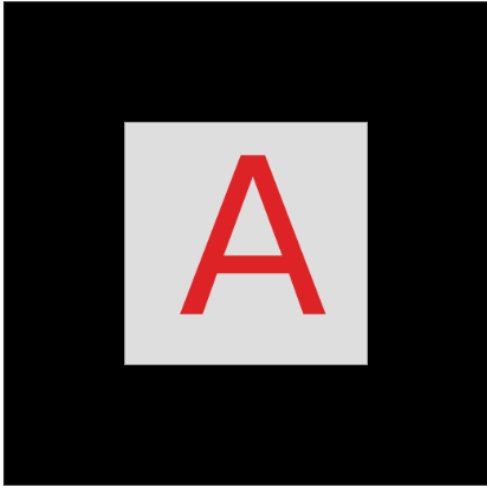
grafeno
