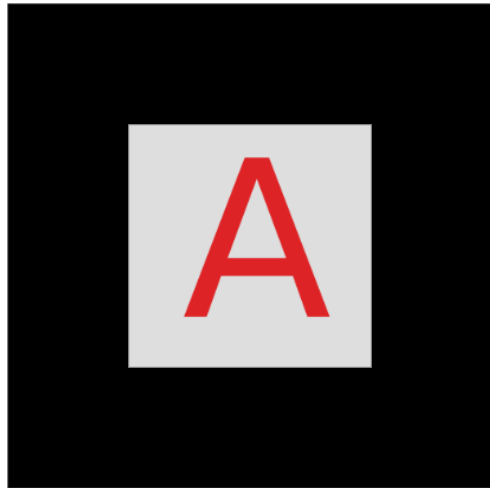
cafeína
