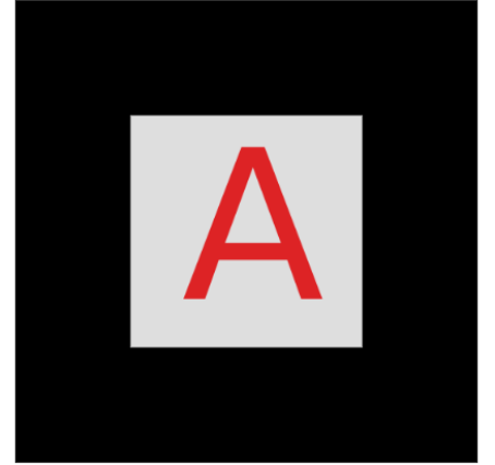
grafeno
