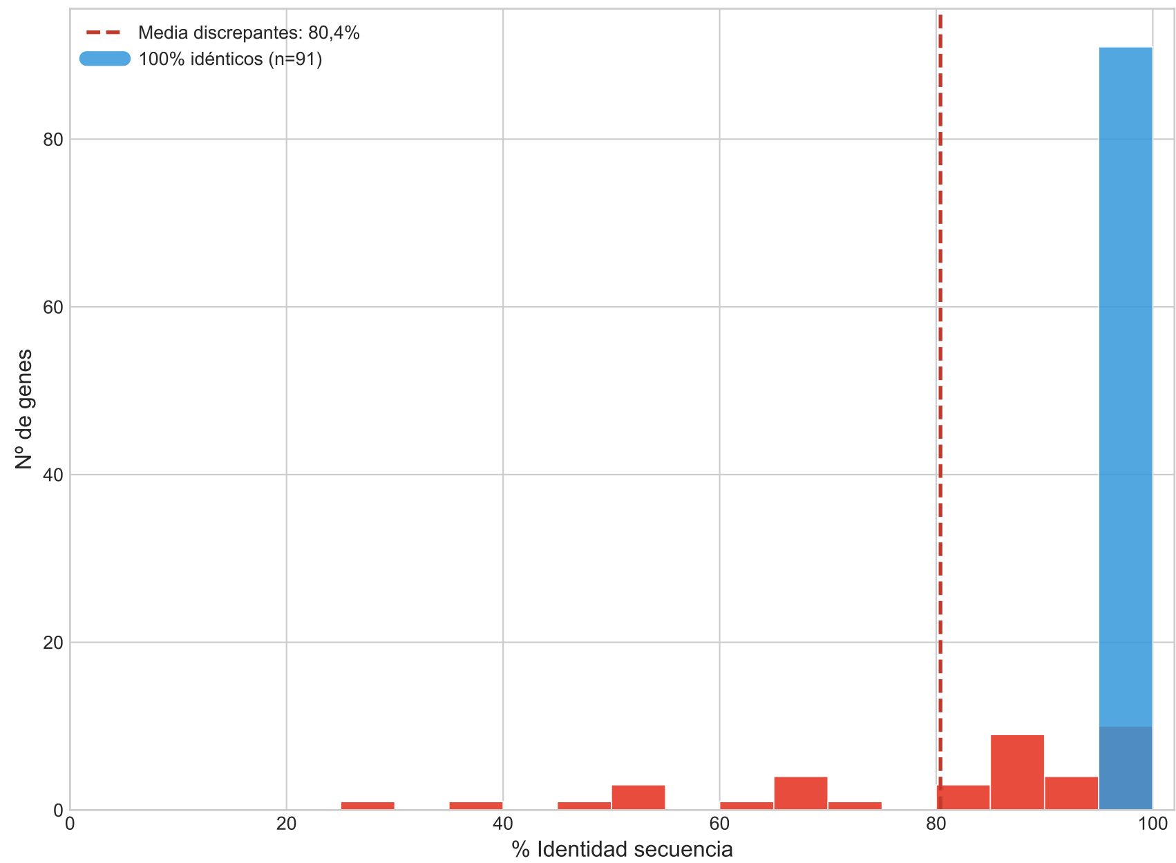
Distribución de identidad (GFF3 vs Exonerate)
