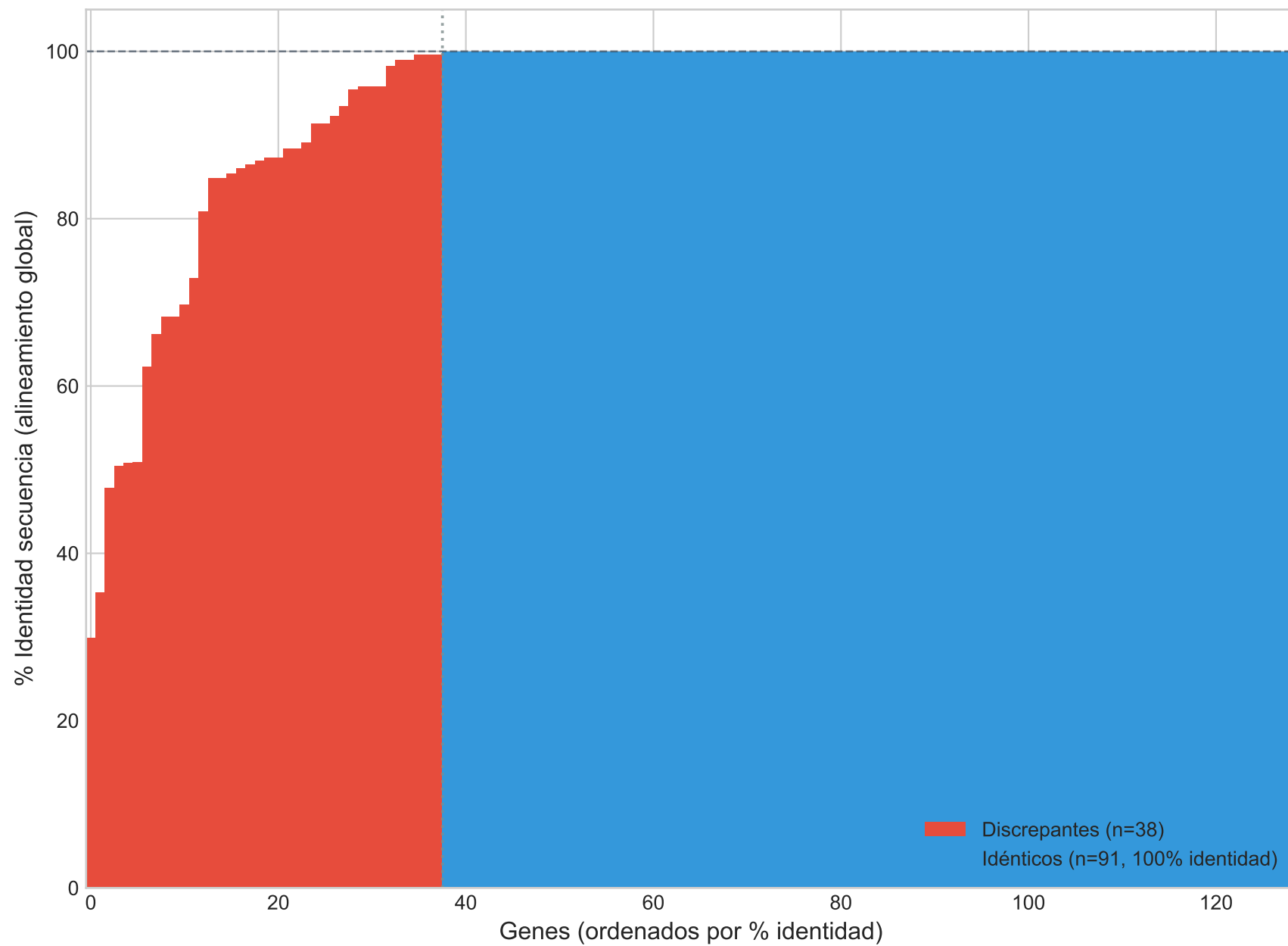
Identidad de secuencia peptídica entre GFF3 y Exonerate por gen de acuaporina
