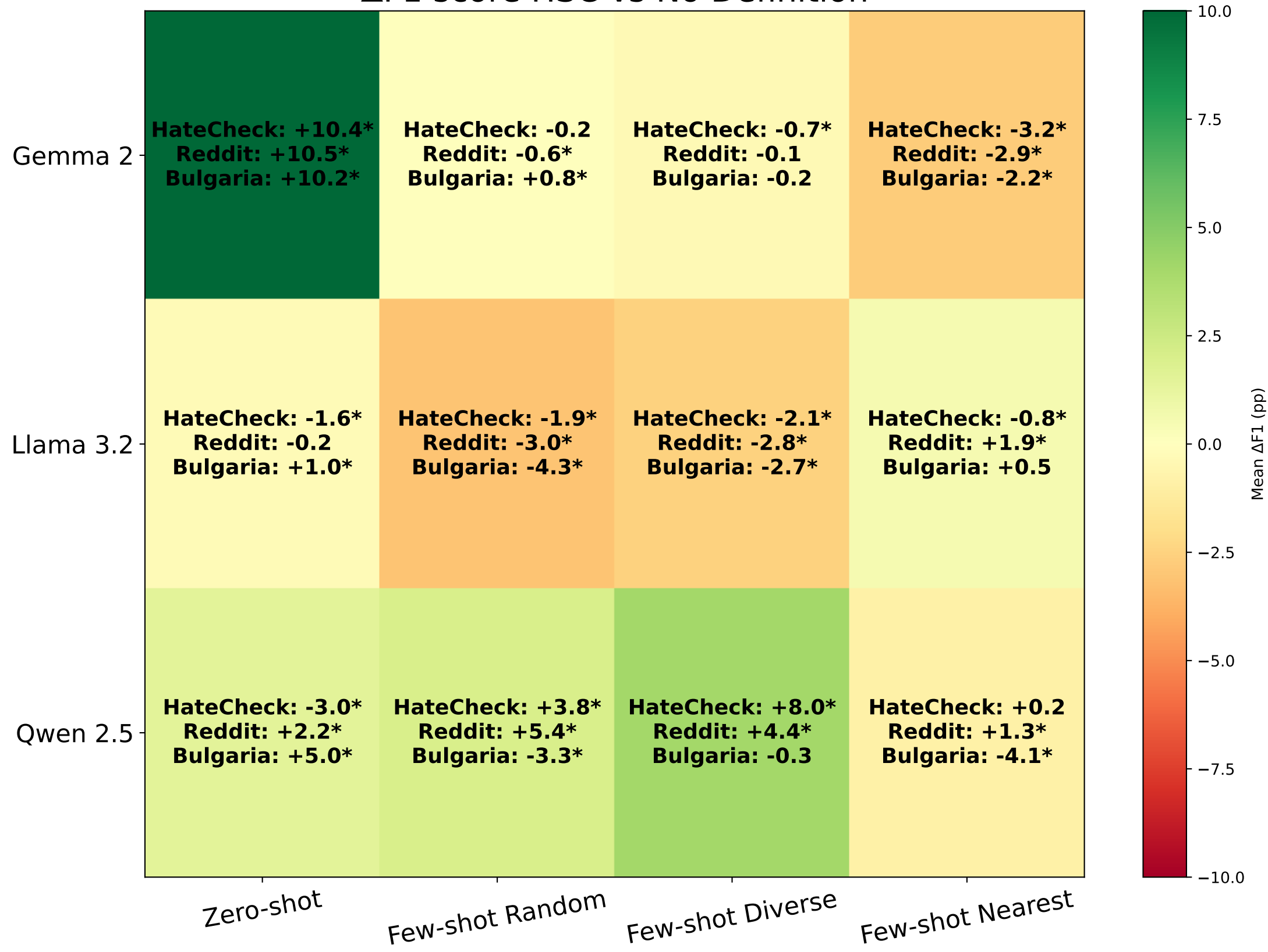
\Delta F1 score HSC vs No Definition
