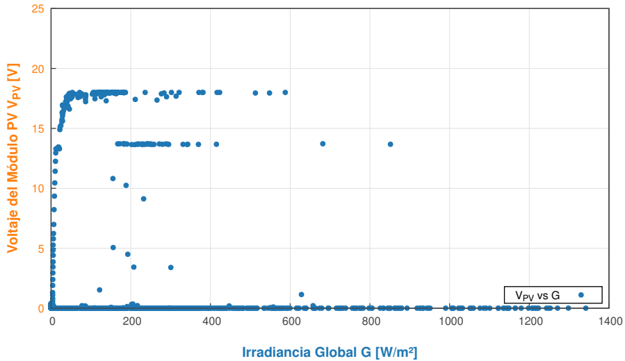
Relación entre Irradiancia Incidente y Voltaje del Módulo PV - 2026-07-16
