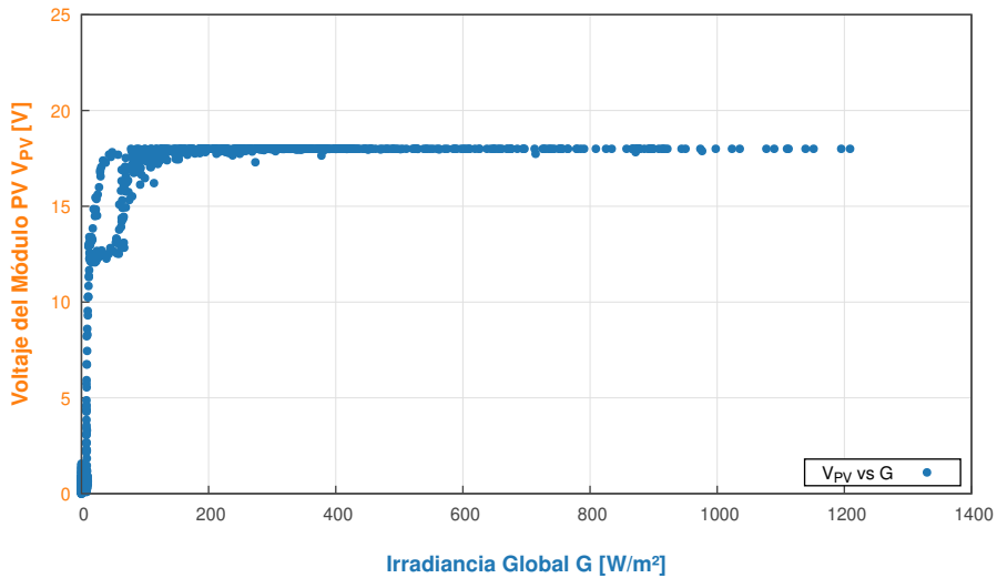
Relación entre Irradiancia Incidente y Voltaje del Módulo PV - 2026-07-17
