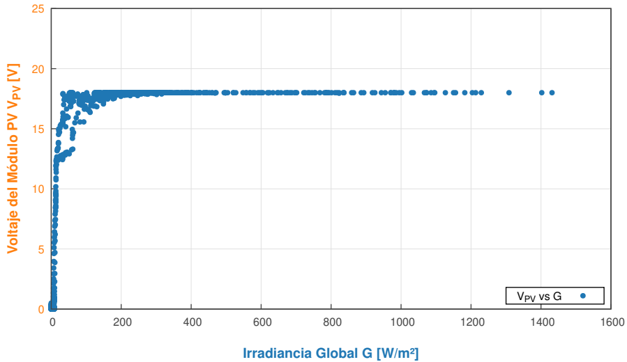
Relación entre Irradiancia Incidente y Voltaje del Módulo PV - 2026-07-18
