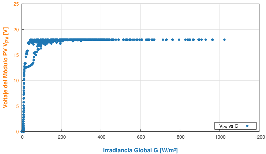
Relación entre Irradiancia Incidente y Voltaje del Módulo PV - 2026-07-19
