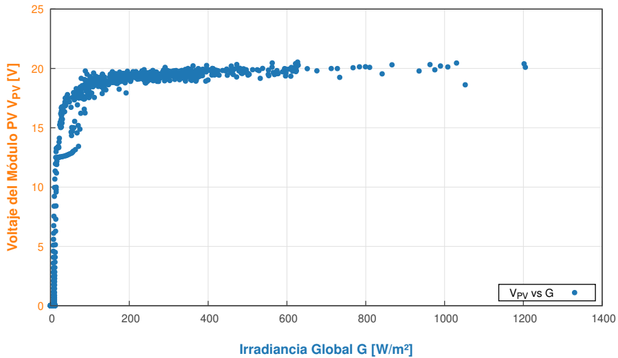
Relación entre Irradiancia Incidente y Voltaje del Módulo PV - 2026-07-22
