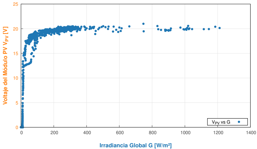
Relación entre Irradiancia Incidente y Voltaje del Módulo PV - 2026-07-23
