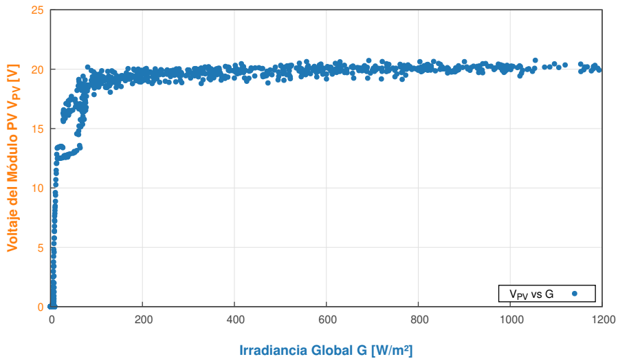
Relación entre Irradiancia Incidente y Voltaje del Módulo PV - 2026-07-24
