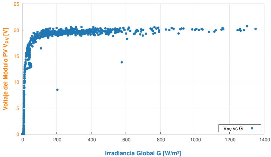
Relación entre Irradiancia Incidente y Voltaje del Módulo PV - 2026-07-25
