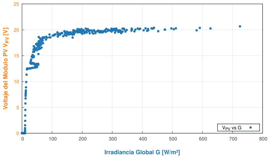
Relación entre Irradiancia Incidente y Voltaje del Módulo PV - 2026-07-26
