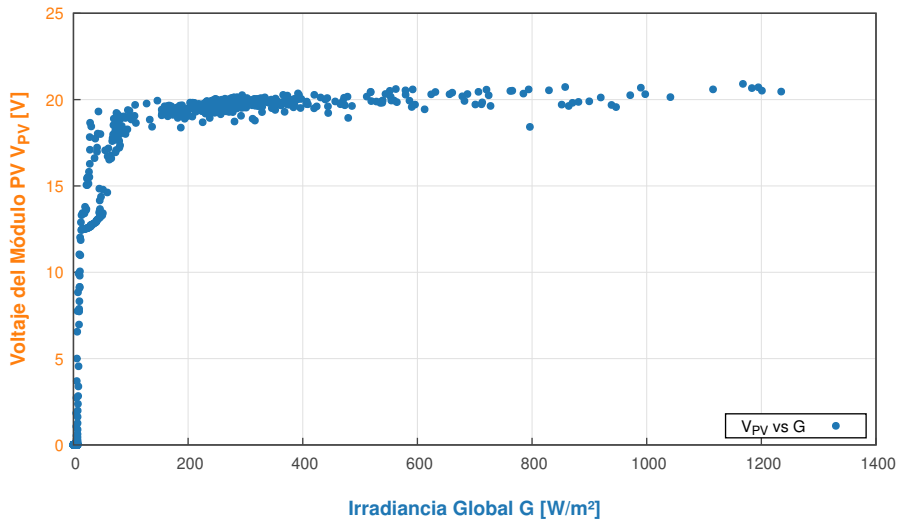
Relación entre Irradiancia Incidente y Voltaje del Módulo PV - 2026-07-27
