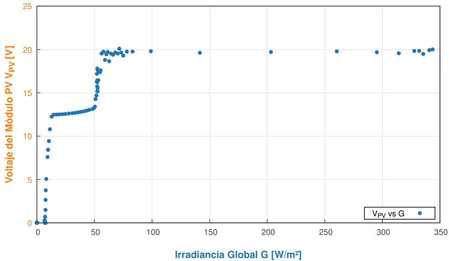
Relación entre Irradiancia Incidente y Voltaje del Módulo PV - 2026-07-28
