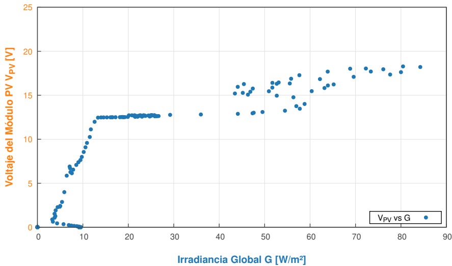
Relación entre Irradiancia Incidente y Voltaje del Módulo PV - 2026-08-08
