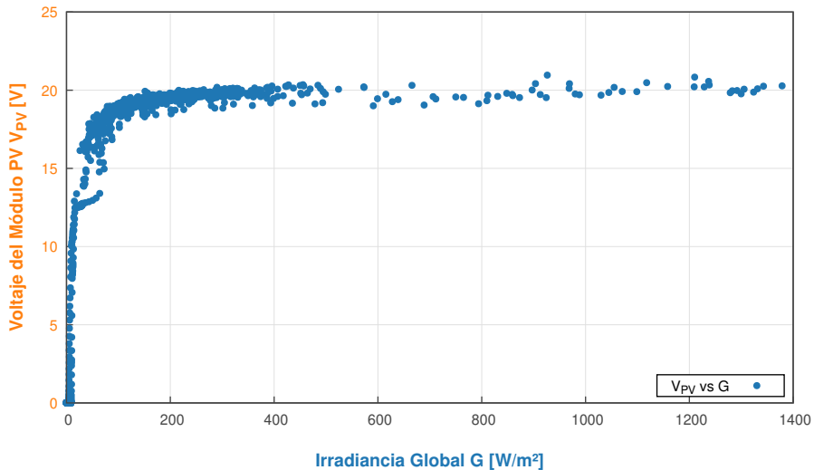
Relación entre Irradiancia Incidente y Voltaje del Módulo PV - 2026-08-09
