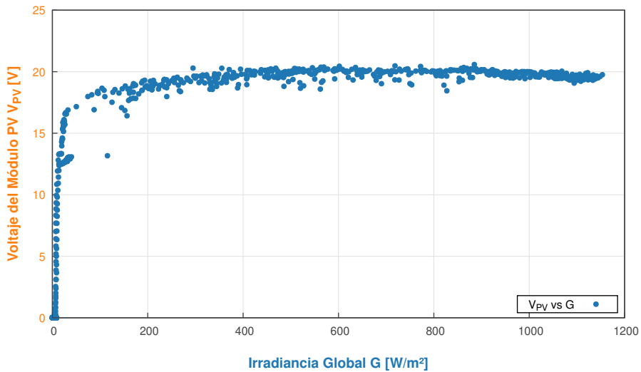
Relación entre Irradiancia Incidente y Voltaje del Módulo PV - 2026-08-10
