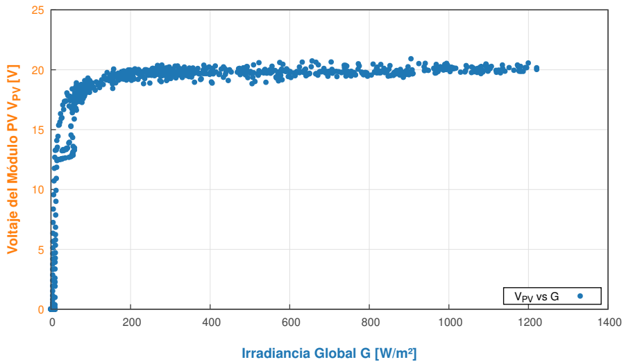
Relación entre Irradiancia Incidente y Voltaje del Módulo PV - 2026-08-12
